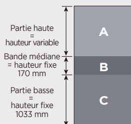
TEMPO H ≥ 2200 mm 1 bande médiane horizontale 3 décors au choix (identiques ou différents)
