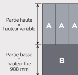
INDUS' H 1300 à 2700 mm L 701 à 1000 mm
